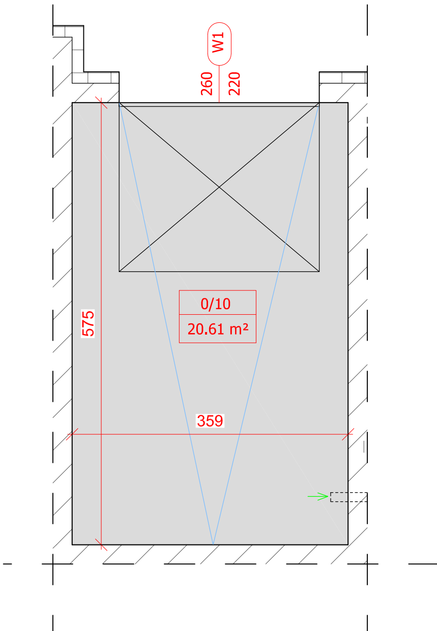
Rzut garażu skala 1:50
